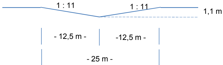
Schnitt C-D
