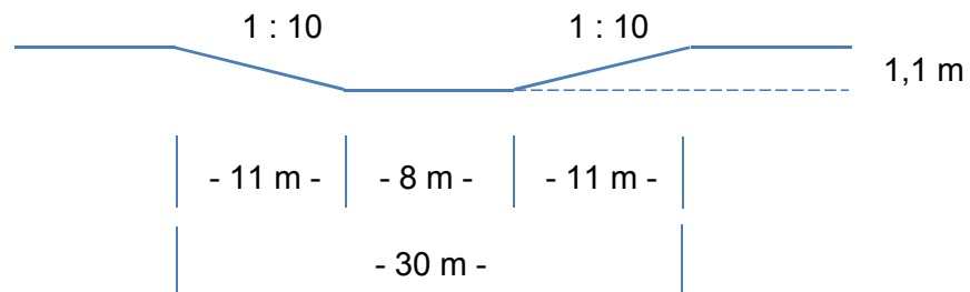
Schnitt A-B
