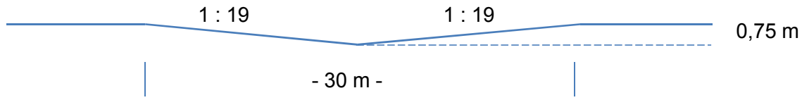
Schnitt A-B
