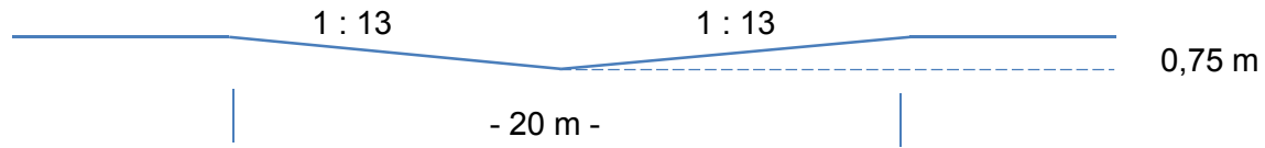
Schnitt C-D
