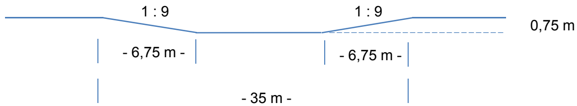
Schnitt A-B
