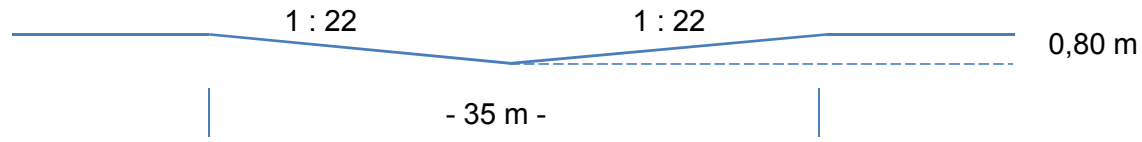
Schnitt A-B
