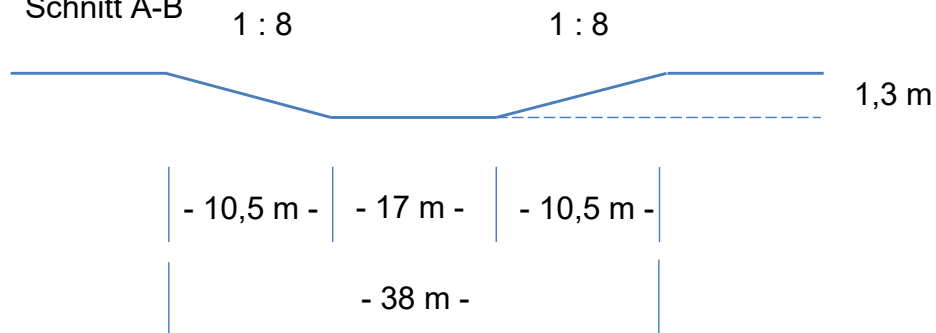
Schnitt A-B
