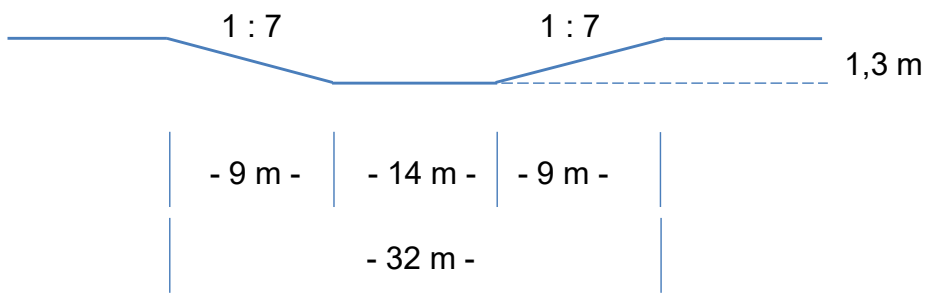
Schnitt A-B
