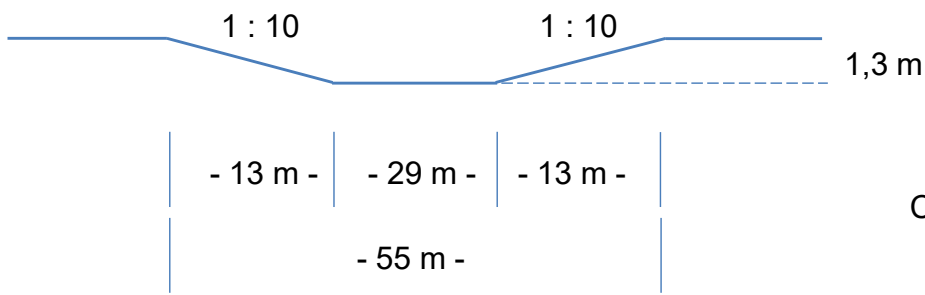
Schnitt A-B
