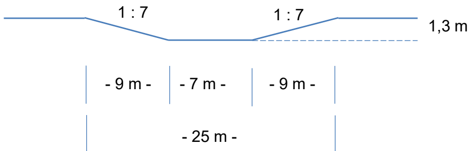
Schnitt C-D
