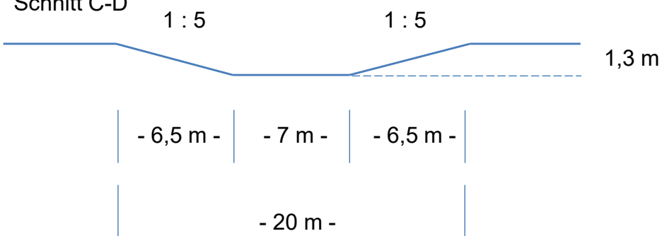
Schnitt C-D
