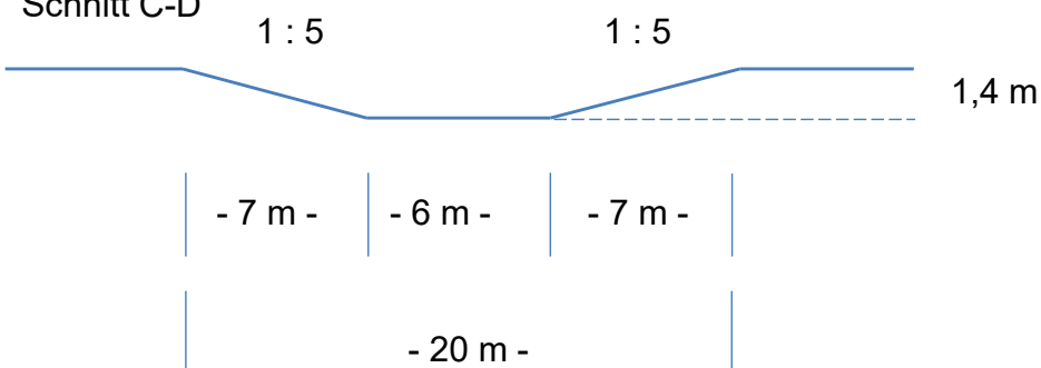
Schnitt C-D
