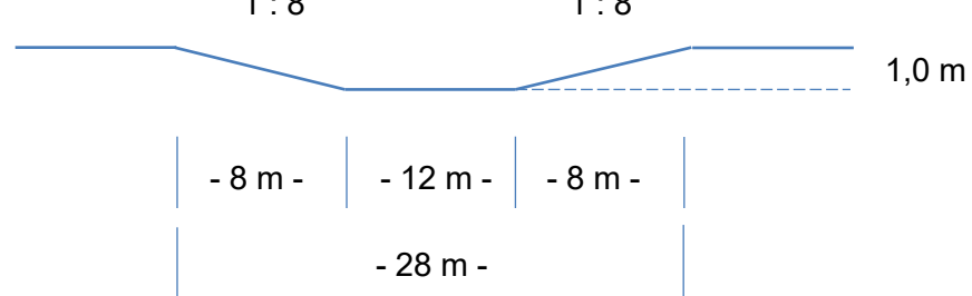
Schnitt A-B
