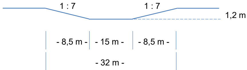
Schnitt A-B
