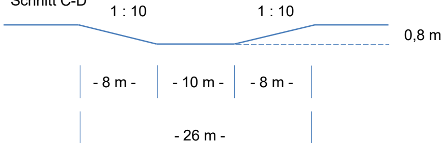
Schnitt C-D
