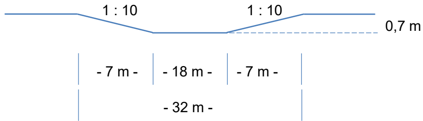
Schnitt A-B
