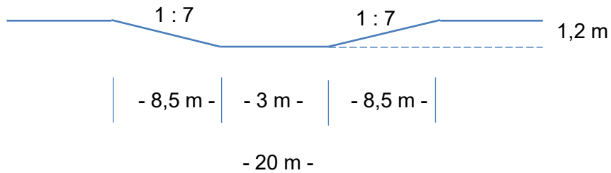
Schnitt C-D
