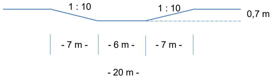
Schnitt C-D
