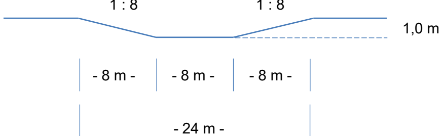
Schnitt C-D
